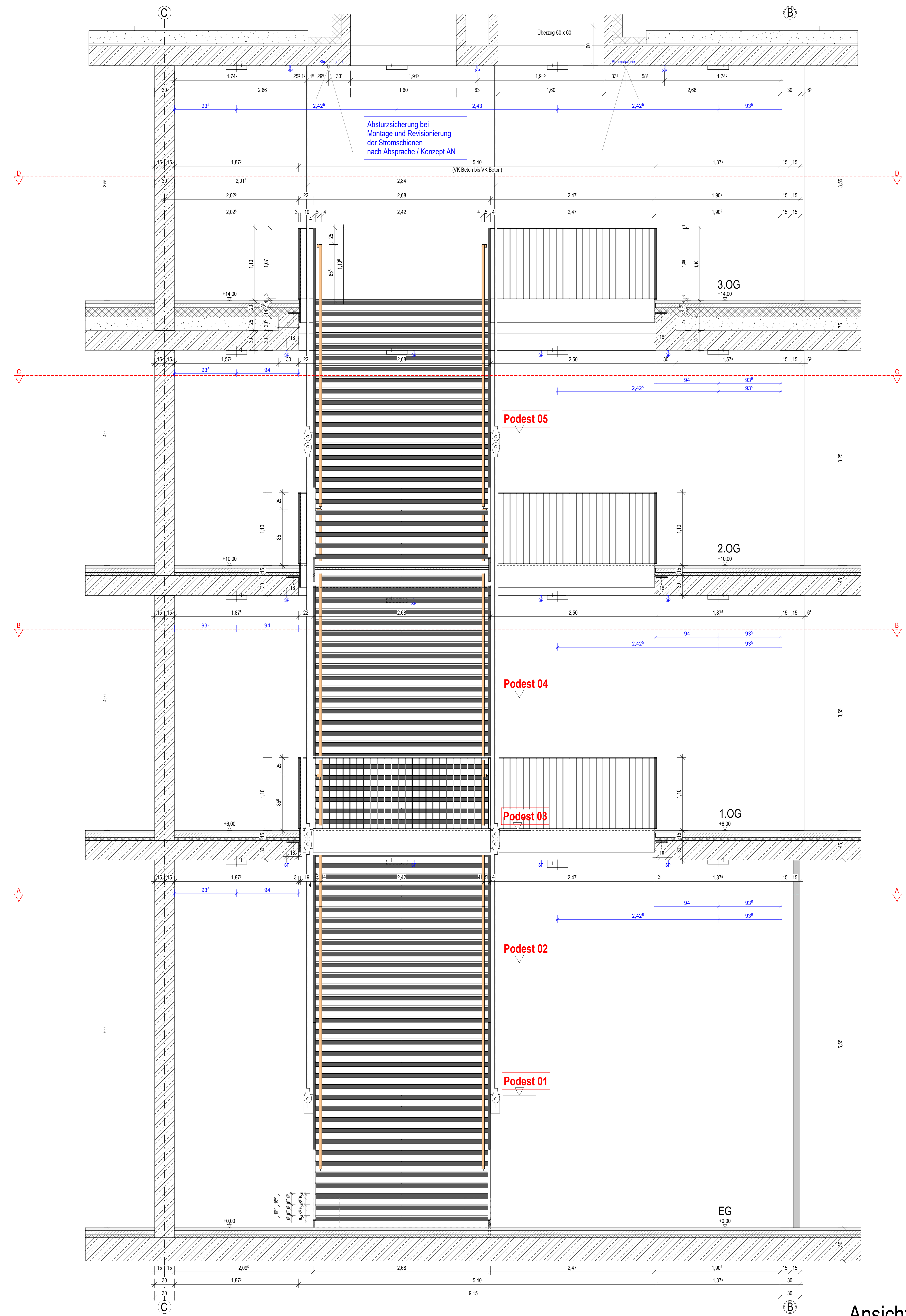
Ansicht 4-4
